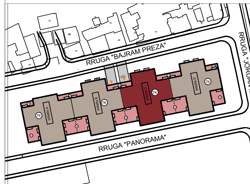
PLANVENDOSJA E OBJEKTIT
